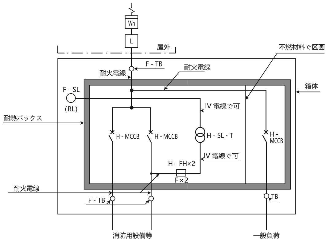
1 電気事業者よりの受電点に使用する場合の例
