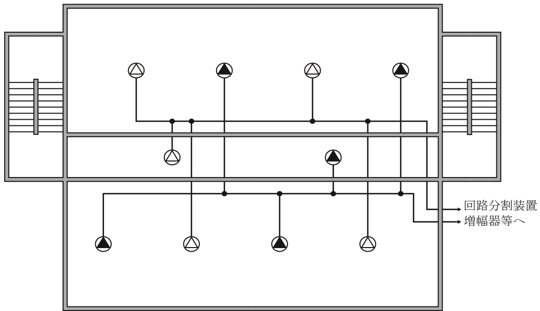
(その 3) 隣接するスピーカーを複数回線化した例
