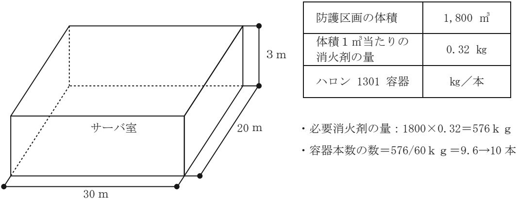
（ハロン 1301 の消火剤の量の算出例）
