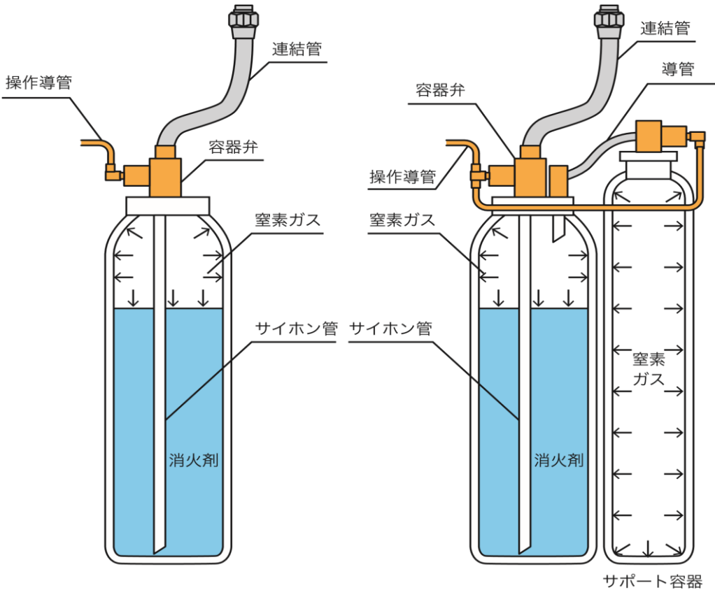
(参考) 蓄圧式の貯蔵容器 ピストンフロー式の貯蔵容器
