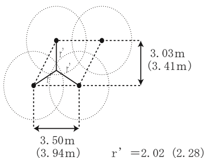
（散水密度が低下しないようにした千鳥型配置の例）
