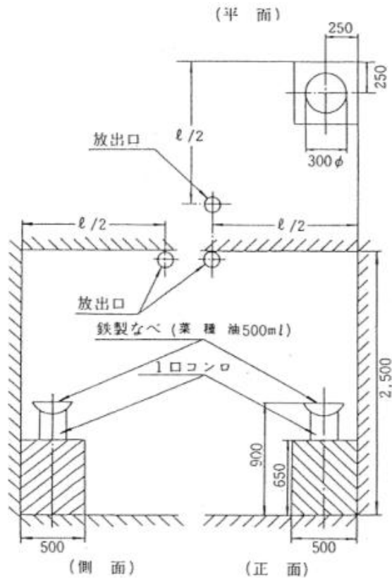
第4 消火試験図
