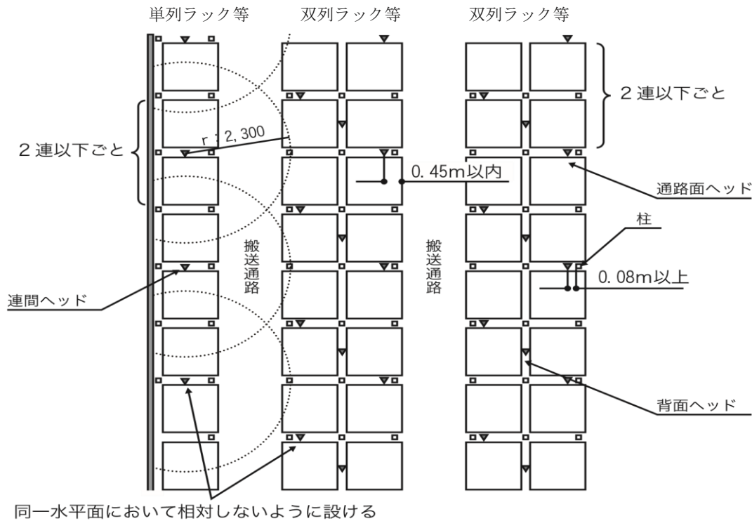
(平面図 レベル1, 3配置)
