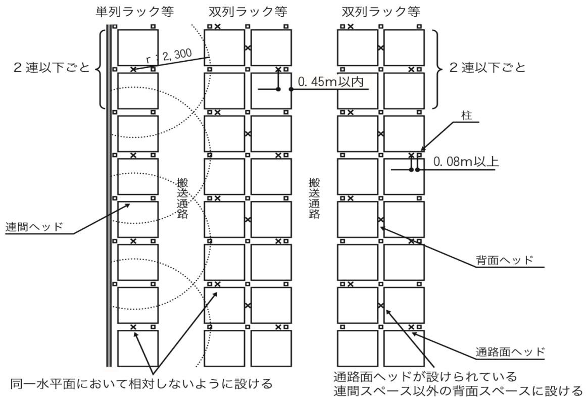
(平面図 レベル1, 3配置)
