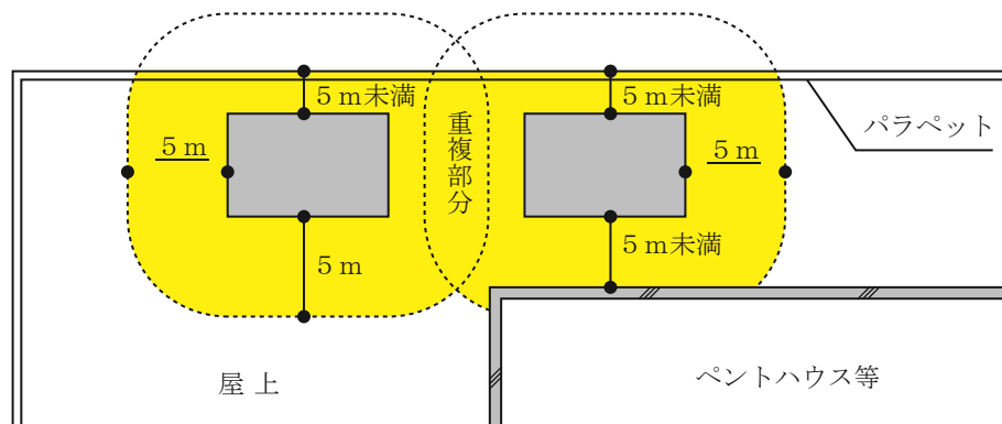
○屋上の場合
