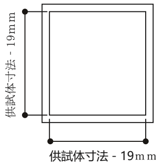
図2 締め枠
