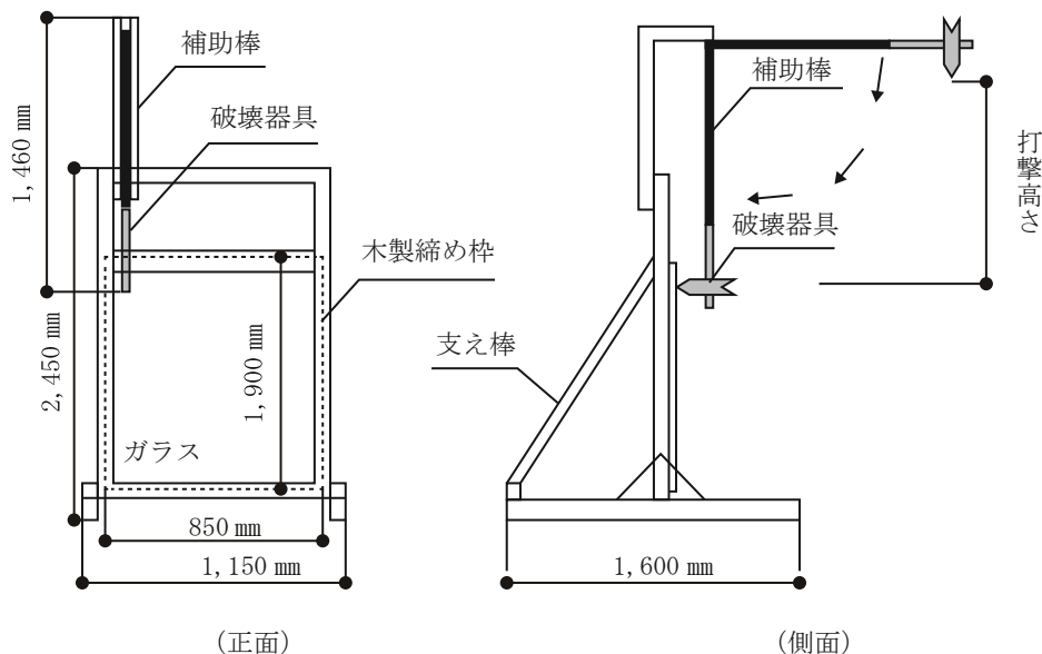
図1 本体
