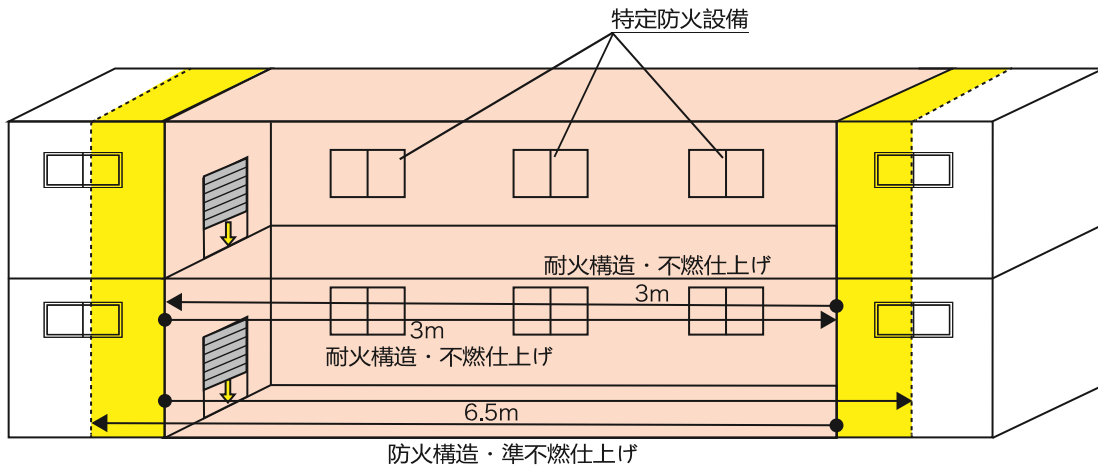
第3-2図 (コアタイプの例)
