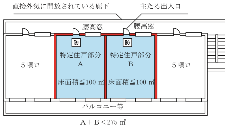
別図6 省令第12条の2第3項
