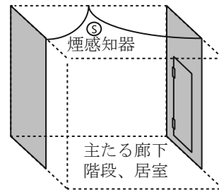
くぐり戸付きの防火戸（特定防火戸）
