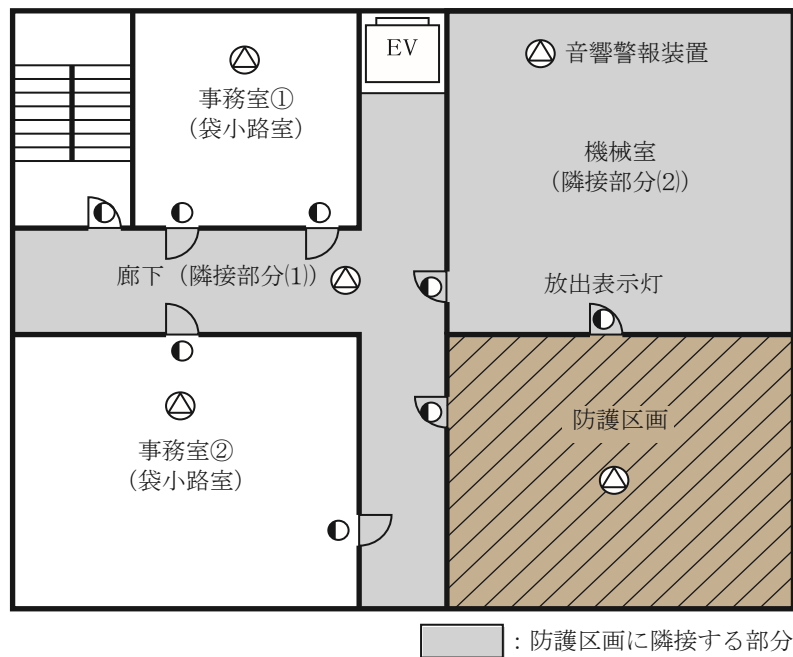
放出表示灯等の設置例(その1)
