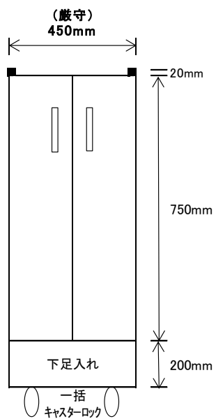
前面
