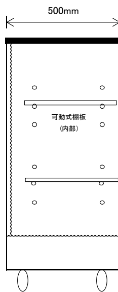
側面(右側)
