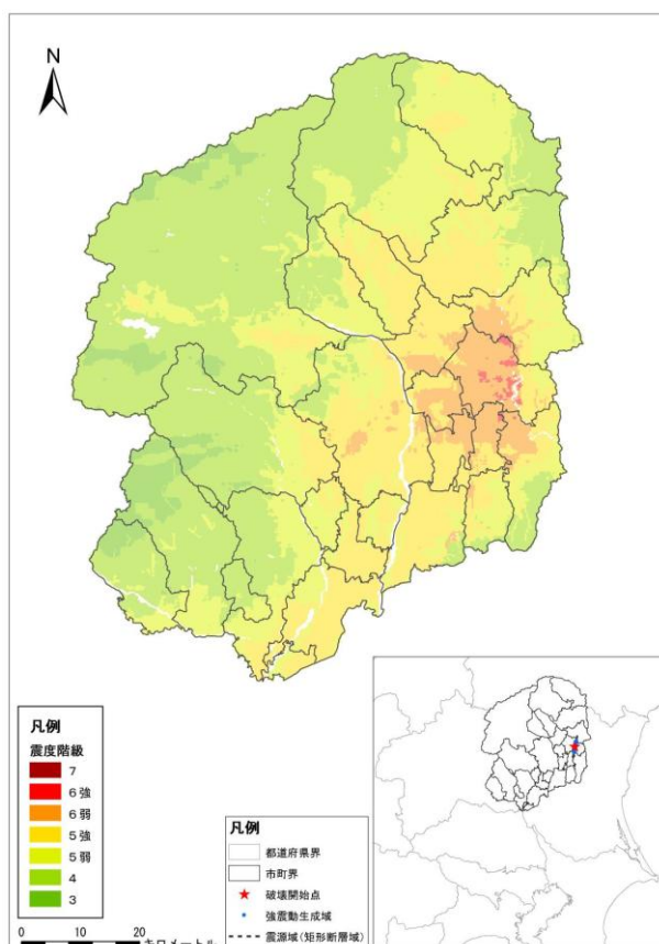
《那須烏山市直下に仮定した震度分布 M6.9》
