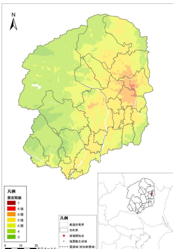
《那珂川町直下に仮定した震度分布 M6.9》
